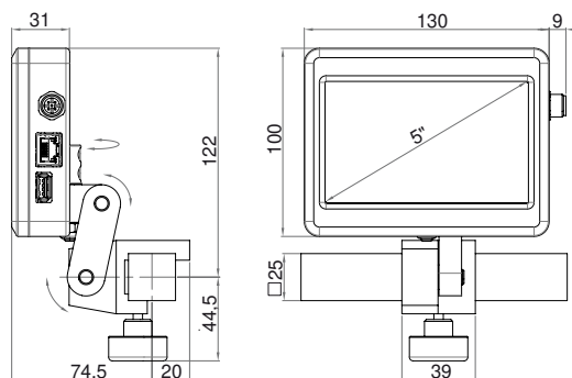
PTS 25 display
