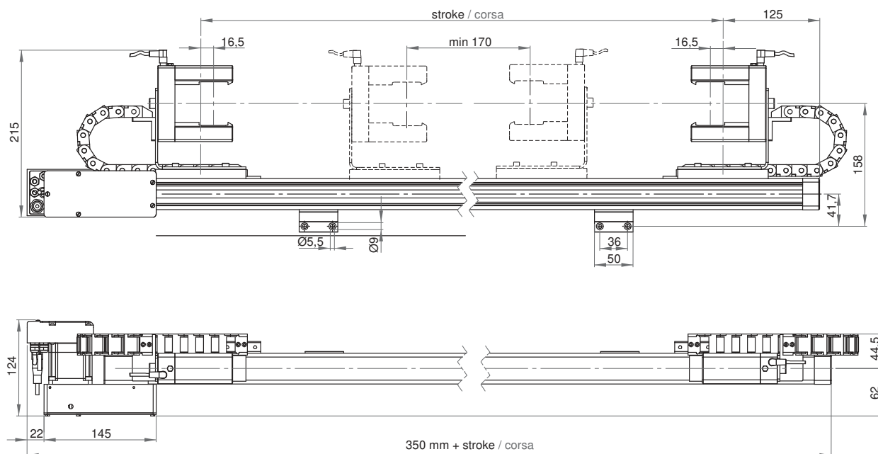
2 sensors - center guide / 2 sensori - guida di centro
