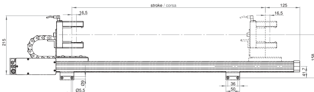
2 sensors - center guide / 2 sensori - guida di centro
